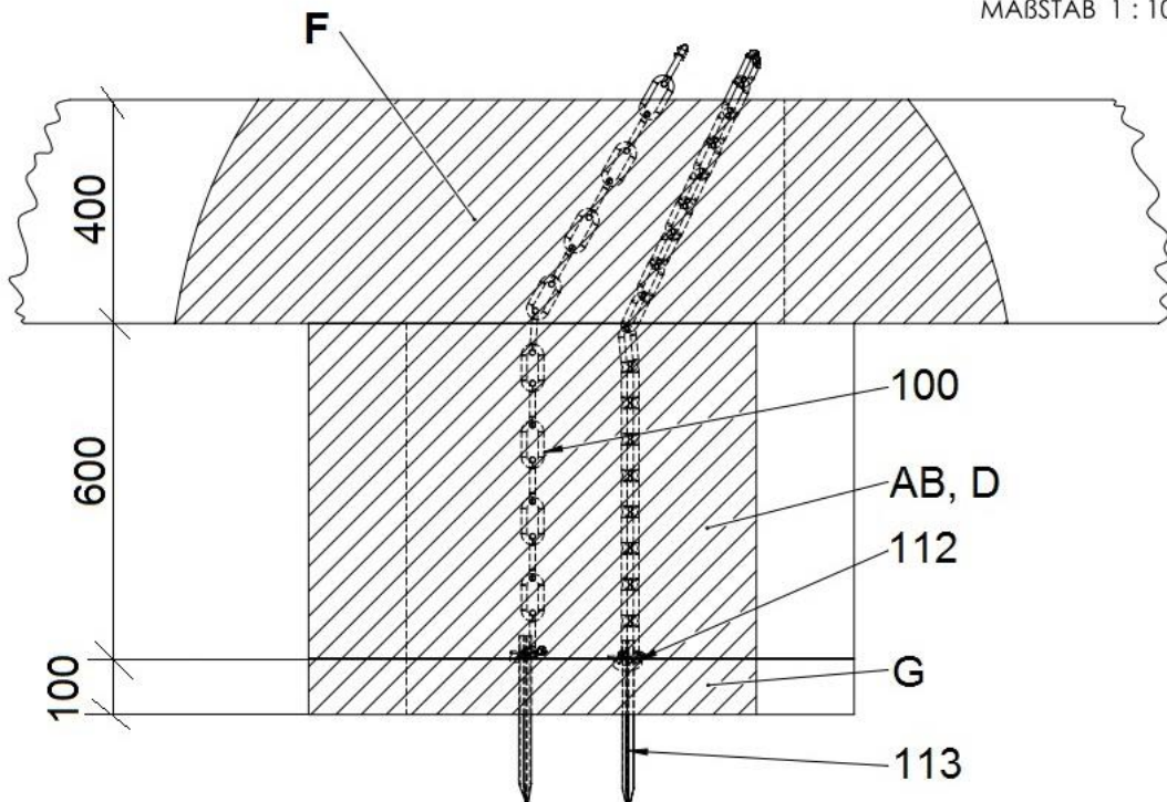
DETAIL MAßSTAB 1 : 10
